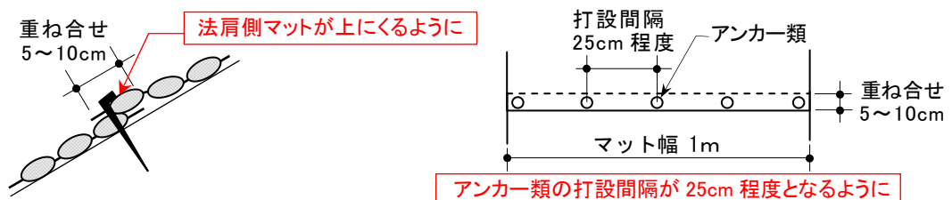
図 1. マット縦方向の重ね合わせとアンカー類の打設
