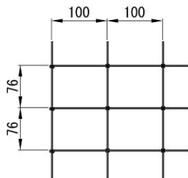
金網目合い詳細図
