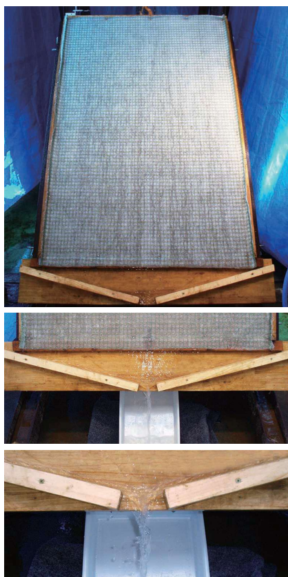
ソイルテクター S 試験雨量 400mm/h
