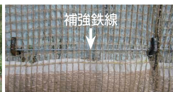
マット内での 補強鉄線の働き
