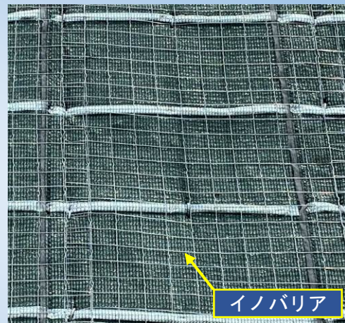
植生マット工との併用事例（試験施工）
