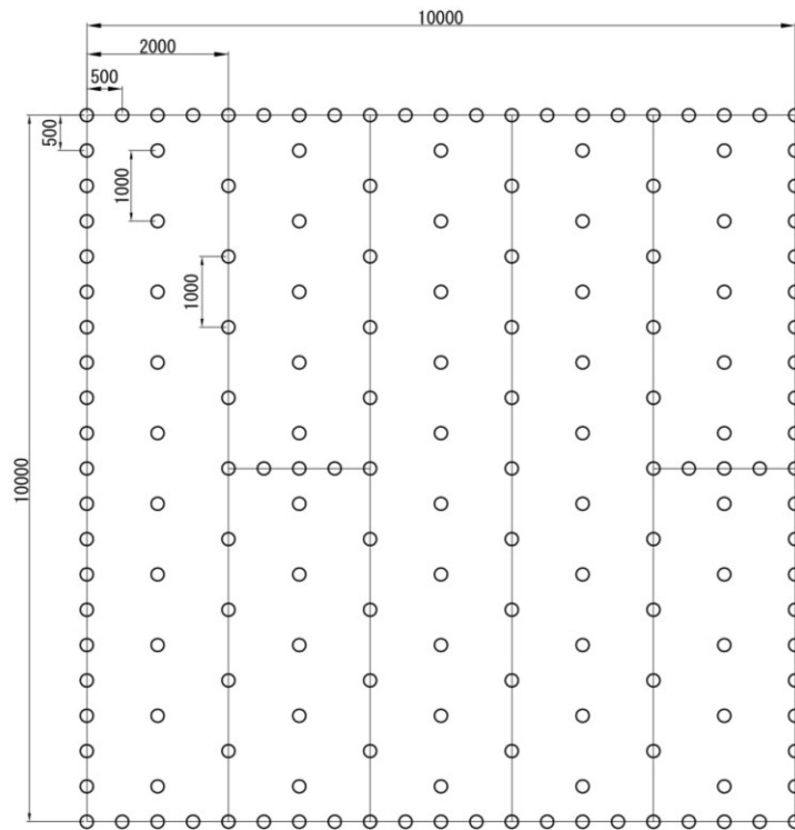
金網目合い詳細図
