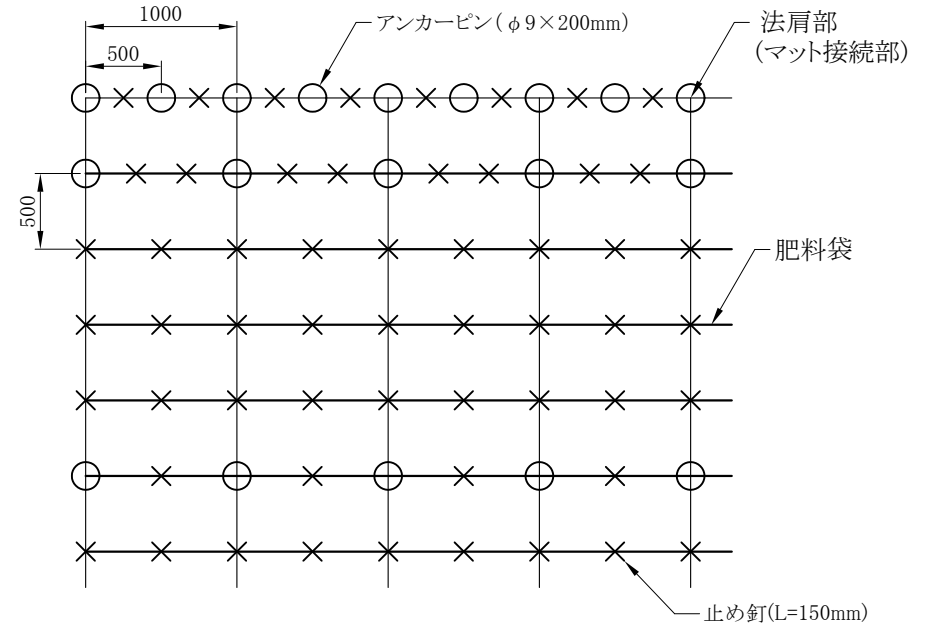
設置打設図
