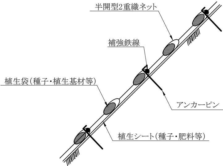
断面図
