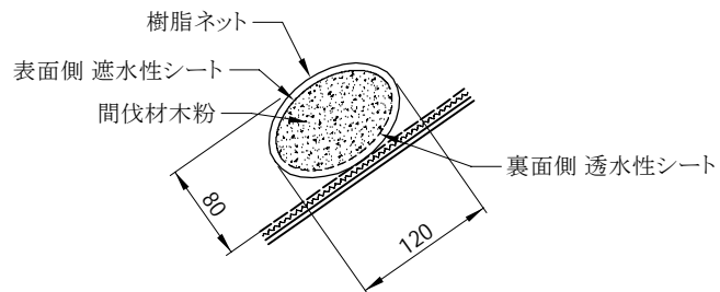
流速軽減袋 詳細図
