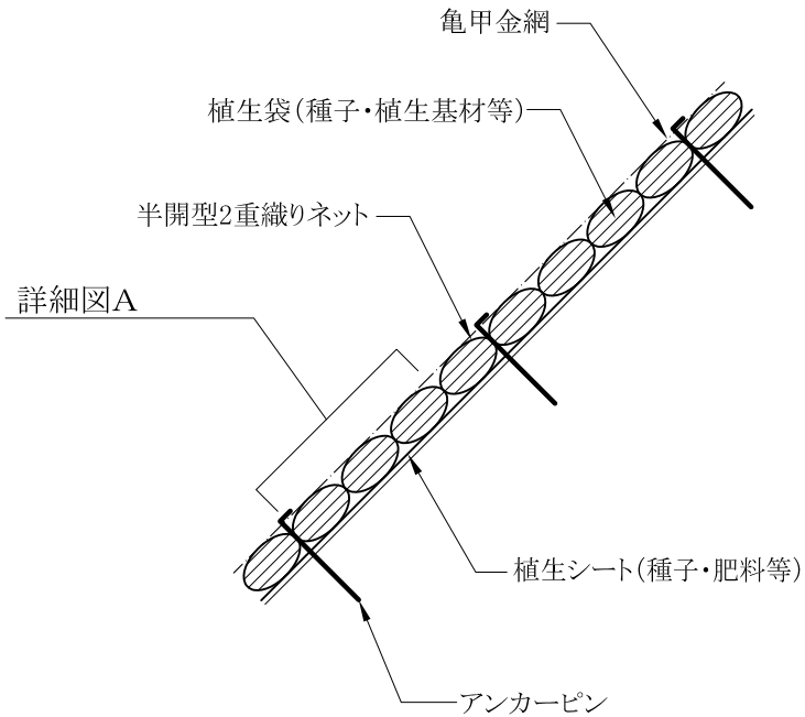
(施工断面図)
