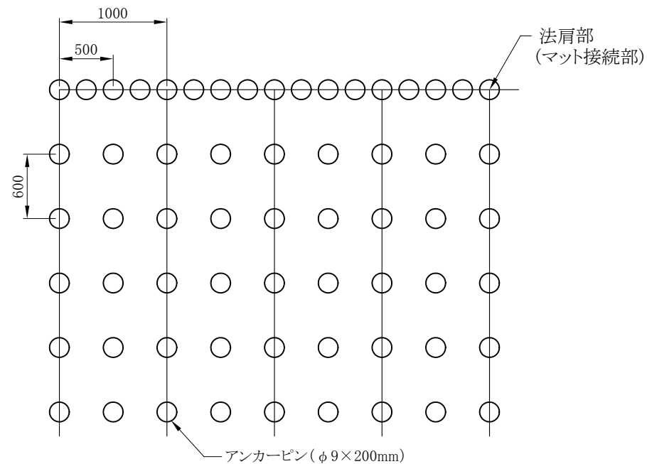
設置打設図
