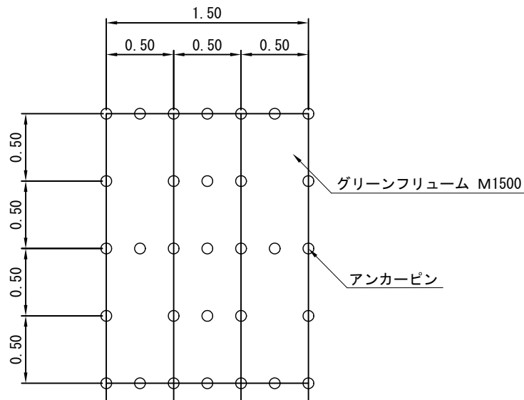
展開図
