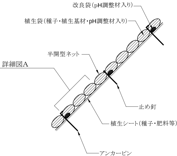
(施工断面図)
