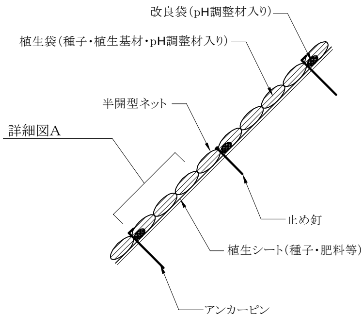
(施工断面図)
