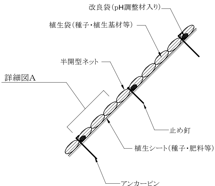
(施工断面図)
