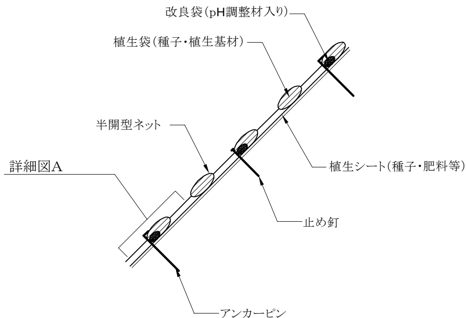
(施工断面図)
