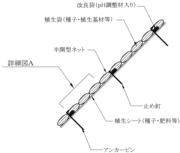
施工断面図
