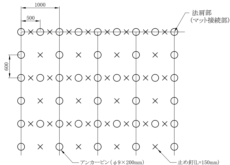
設置打設図
