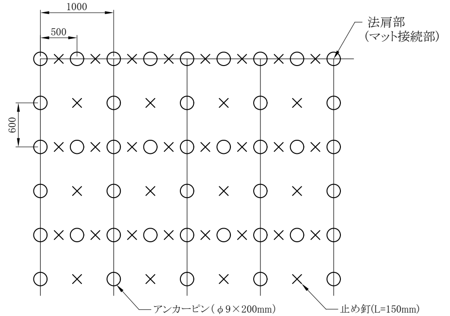
設置打設図
